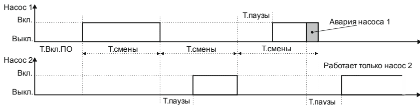
Рисунок 3.1 - Диаграмма переключения насосов
