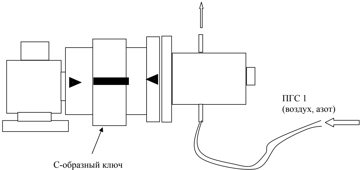
Рисунок Г.1 – Схема регулировки «нуля» преобразователя
